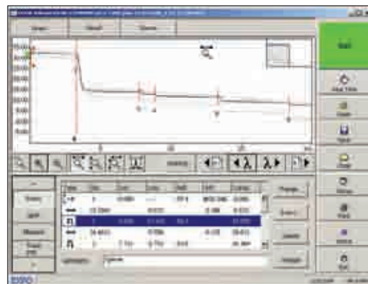
Рефлектометр FTB-7300D с легкостью проводит измерения линии с разветвителями с большим количеством портов и высокими значениями потерь.
