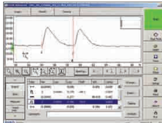
Мертвая зона по затуханию в рефлектометре FTB-7000D позволяет ему полноценно провести измерения типичного стационарного кабеля длиной всего пять метров с коннекторами UPC (отражения ниже -55 дБ).
